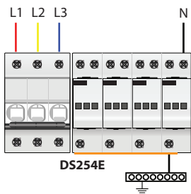
Sơ đồ đấu nối 2
