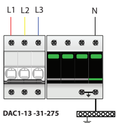
Sơ đồ đấu nối 1
