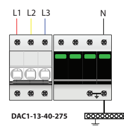
Sơ đồ đấu nối 2
