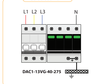
Sơ đồ đấu nối 2
