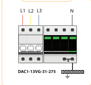
Sơ đồ đấu nối 1
